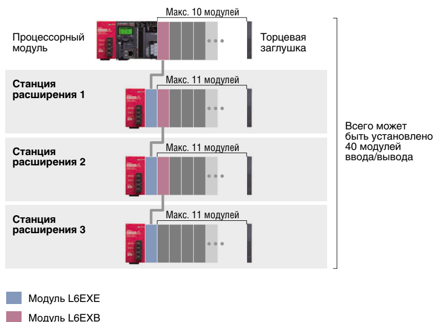
Конструктив без шасси позволяет экономить пространство в шкафу управления
