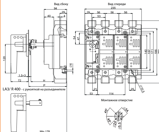
LA3/ D 400 - с ручкой на дверцу шкафа
