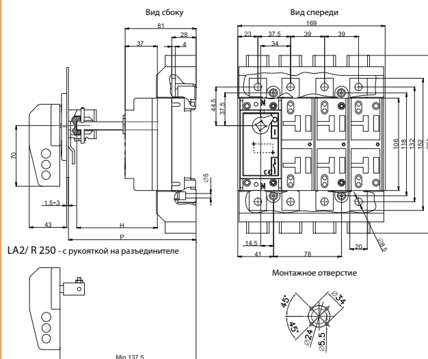
LA2/ D 250 - с ручкой на дверцу шкафа
