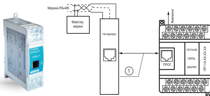
Схема підключення ПР-МИ485 до ОВЕН ПР110/114 та мережі RS-485 - кабель «КС8»
