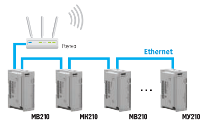
Підключення модулів Mx210 до хмарного сервісу
