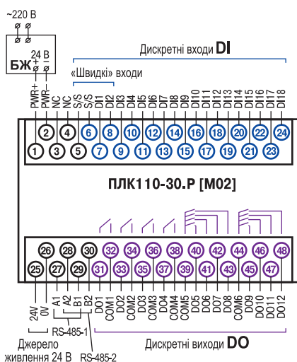
Схема розташування та призначення клем ПЛК110-24.30.Р [M02]
