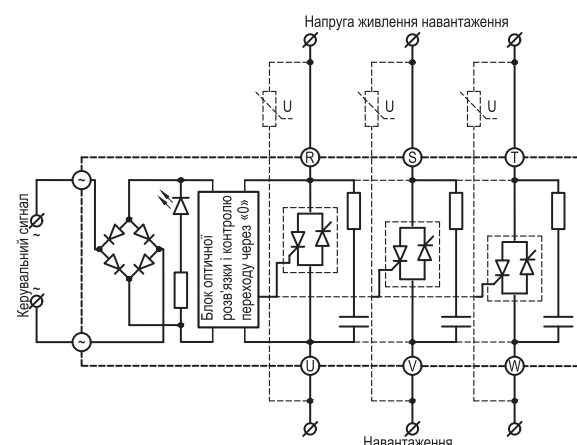
Схема вмикання серії HT-xx44.ZA2 (виходи – тиристори)
