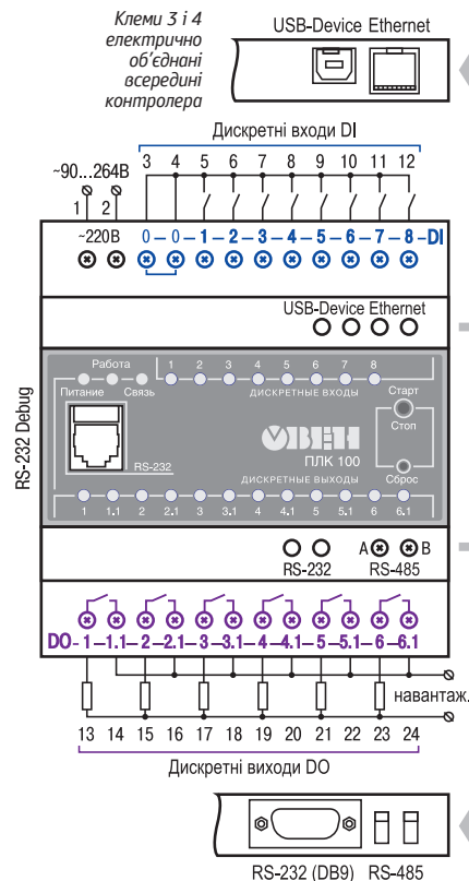
Схема підмикання ПЛК100-220.Р
