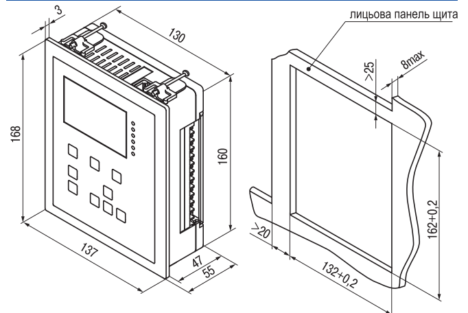
Габаритний кресленник ПЛК73 у корпусі щитового кріплення
