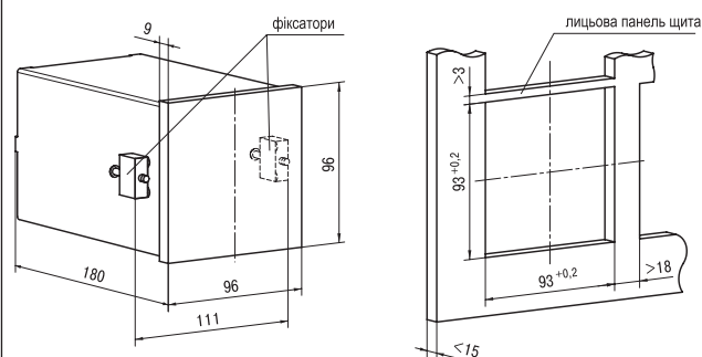
Щ — корпус щитового кріплення габаритні розміри: 96х96х180 мм, ступінь захисту з боку передньої панелі IP20
