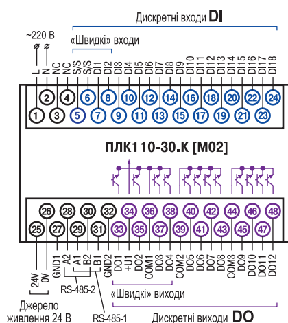
Схема розташування та призначення клем ПЛК110-220.30.К [M02]
