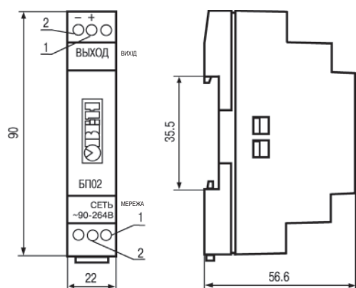
Д1 — корпус для кріплення на DIN-рейку габаритні розміри: 22х90х56,6 мм ступінь захисту з боку передньої панелі IP20
