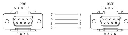
Кабель КС4 для підмикання ПЛК110 до панелей ИП320, СП270 та СП3хх (порт RS-232 Download)
