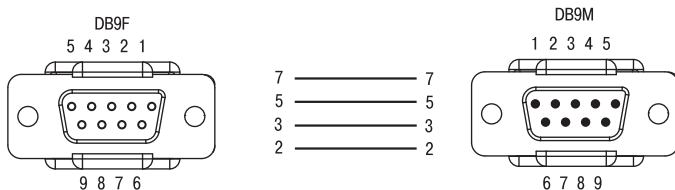
Схема кабелю подовжувального КС5
