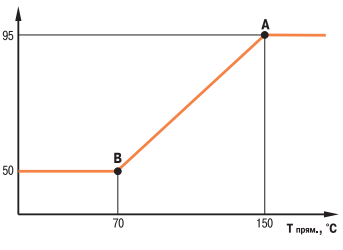
Приклад графіка температури зворотної води — T_{зв.мах.} = f(T_{прям.})
