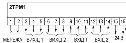
Схема розташування та призначення клем 2TRM1
