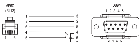
Схема кабелю КС3 «ПЛК-Модем»
