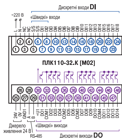
Схема розташування та призначення клем ПЛК110-220.32.К [M02]
