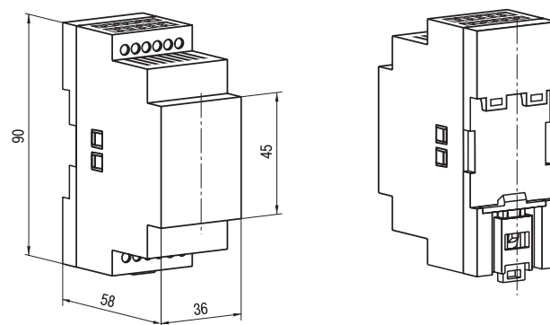
Д2 — корпус для кріплення на DIN-рейку 35 мм габаритні розміри: 36х90х58 мм ступінь захисту з боку передньої панелі IP20
