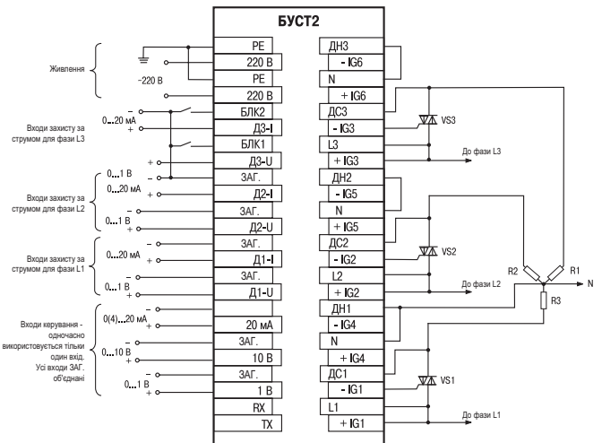
Схема з'єднання для типу підмикання навантаження «зірка з нейтраллю та симісторами»
