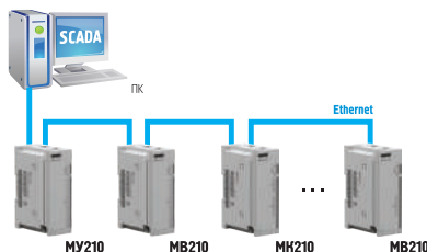
Підключення модулів Mx210 до ПК зі SCADA-системою для віддаленого вводу/виводу сигналів
