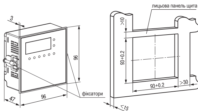
Щ11 — корпус щитового кріплення габаритні розміри: 96х96х49 мм, ступінь захисту з боку передньої панелі IP54
