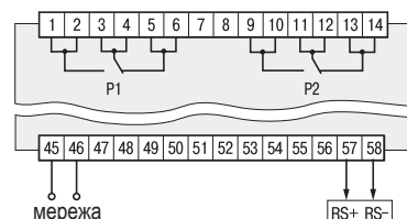
Схема підмикання вихідних реле
