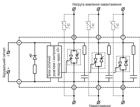
Схема вмикання серії HT-xx44.ZD3 (виходи – симістори (TRIAC))
