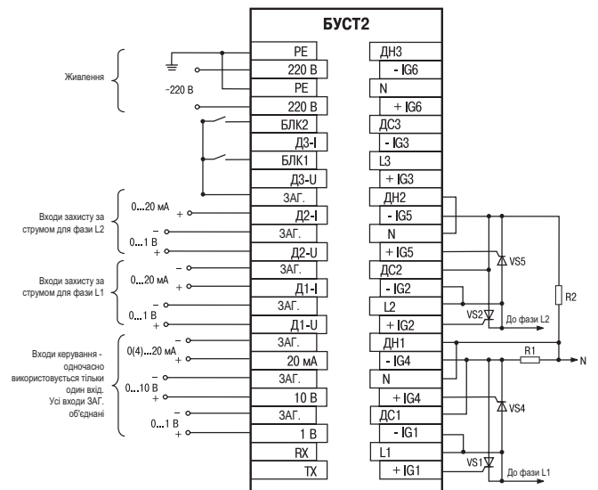
Схема з'єднування для типу підмикання навантаження «дві фази, 220 В»
