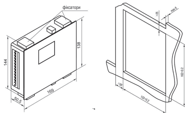
Щ7 — корпус щитового кріплення габаритні розміри: 169х138х50 мм, ступінь захисту з боку передньої панелі IP54
