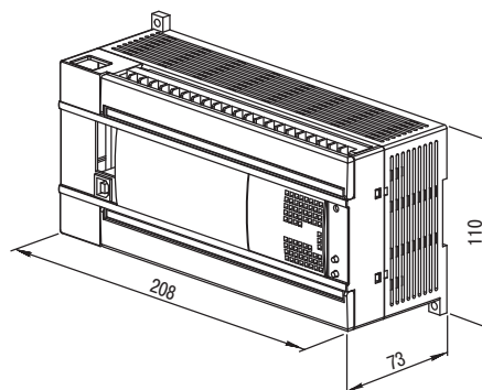
Габаритний кресленик корпусу ПЛК110-60[M02]
