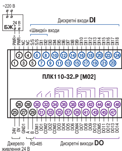
Схема розташування та призначення клем ПЛК110-24.32.Р [M02]
