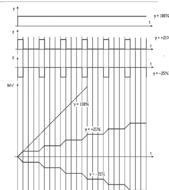
Графік сигналів на виході ШІМ та ВМ при керуванні середньою швидкістю регульовального впливу \gamma
