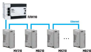
Підключення модулів Mx210 до ПЛК за топологією «ланцюжок» (Daisy Chain)
