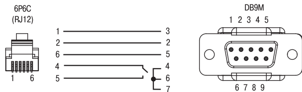
Схема кабелю КС3 для підмикання модему до ПЛК100 за інтерфейсом RS-232
