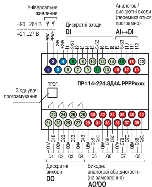
Схема розташування та призначення клем PR114
