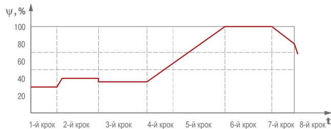
Графіки температури та вологості встановленого температурно-вологісного режиму.
