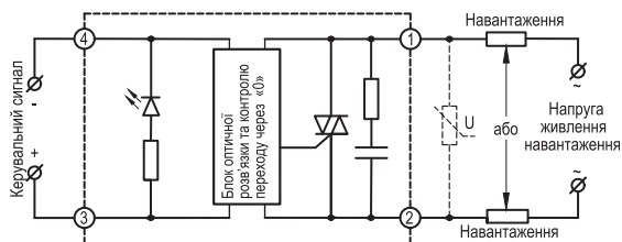
Схема вмикання серії MD-xx44.ZD3
