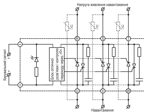
Схема вмикання серії HT-xx44.ZD3 (виходи – тиристори)
