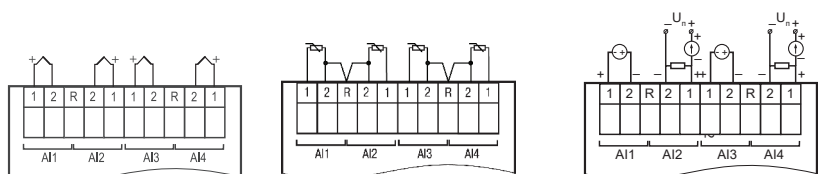
Схеми підм'якання аналогових входів до ПРМ-х.3
