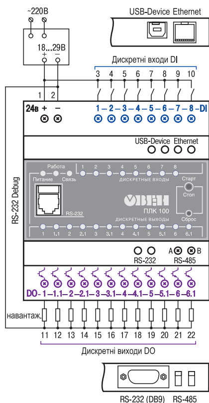
Схема підмикання ПЛК100-24.К
