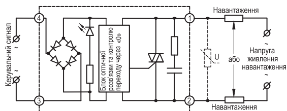
Схема вмикання серії HD-xx44.ZA2 (вихід – симістор (TRIAC))
