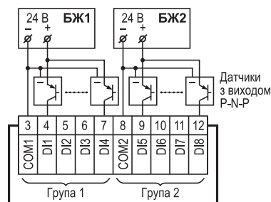
Схема підмикання датчиків, що мають на виходу транзистор р-п-р-типу з відкритим колектором
