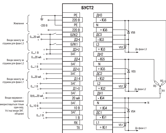
БУСТ2 Живлення Входи захисту за струмом для фази L3 Входи захисту за струмом для фази L2 Входи керування - одночасно використовується тільки один вхід. Усі входи 3АГ, об'єднані ДН3 ДС3 Л3 ДН2 ДН1 ДС1 Л1 VS3 VS2 VS1 До фази L3 До фази L2 До фази L1 PE 220 В PE 220 В БЛК2 ДЗ-І БЛК1 ДЗ-ІІ 3АГ. Д2-І 3АГ. Д2-ІІ 3АГ. Д1-І 3АГ. Д1-ІІ 3АГ. 20 мА 3АГ. 10 В 3АГ. 1 В RX TX - 220 В 0...20 мА + 0...1 В - 0...20 мА + 0...1 В - 0(4)...20 мА + 0...10 В + 0...1 В + - IG6 N + IG6 - IG3 + IG3 - IG5 N + IG5 - IG2 L2 + IG2 - IG4 N + IG4 - IG1 + IG1 R3 R2 R1
