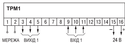
Схема розташування та призначення клем TRM1
