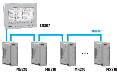
Підключення модулів Mx210 до панелі оператора СП307-Р з інтерфейсом Ethernet
