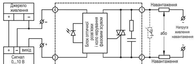
Схема вмикання серії HD-xx22.10U
