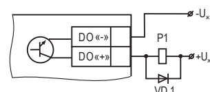
Схема підмикання вихідного пристрою
