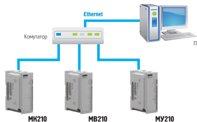
Підключення модулів Mx210 до ПЛК за топологією «зірка»
