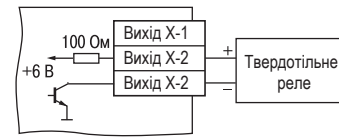
Вихідний елемент типу Т (для керування твердотільним реле)
