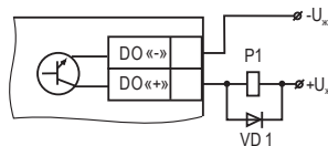
Схема підмикання вихідного пристрою
