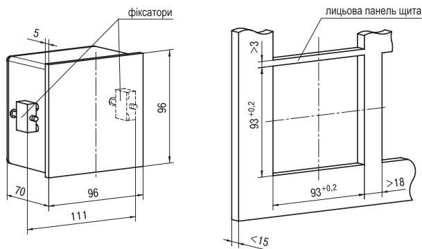
Щ1 — корпус щитового кріплення габаритні розміри: 96х96х70 мм, ступінь захисту з боку передньої панелі IP54
