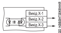
Вихідний елемент типу С (симісторна оптопара)
