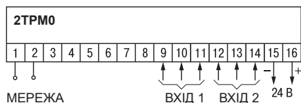
Схема розташування та призначення клем 2TRM0
