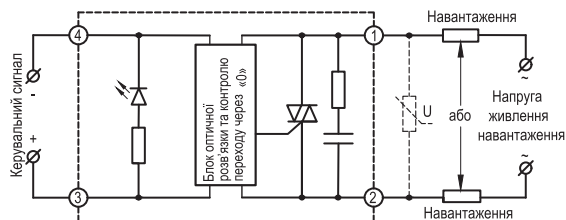
Схема вмикання серії HD-xx44.ZD3
