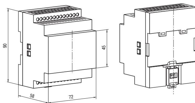
Д4 — корпус для кріплення на DIN-рейку 35 мм габаритні розміри: 72х90х58 мм, ступінь захисту з боку передньої панелі IP20
