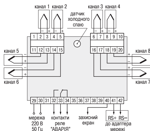
Схема підмикання пристрою модифікації УКТ38-В.04 з термоелектричними перетворювачами типу ТХК(Л), ТХА(К)
