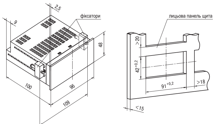
Щ2 — корпус щитового кріплення габаритні розміри: 96х48х100 мм ступінь захисту з боку передньої панелі IP54
