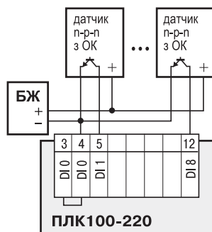
ПЛК100-220, датчик п-р-п-типу
