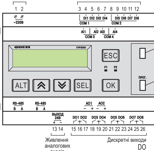
Схема розташування та призначення клем ПР200
