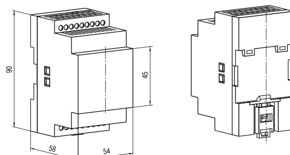
Д3 — корпус для кріплення на DIN-рейку 35 мм, габаритні розміри: 54х90х58 мм ступінь захисту з боку передньої панелі IP20
