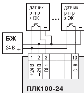
ПЛК100-24, датчик р-р-п-типу
