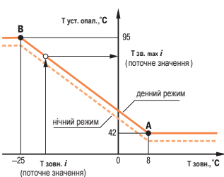
Приклад опалювального датчика — T_{уст.опал.} = f(T_{зовн.})
