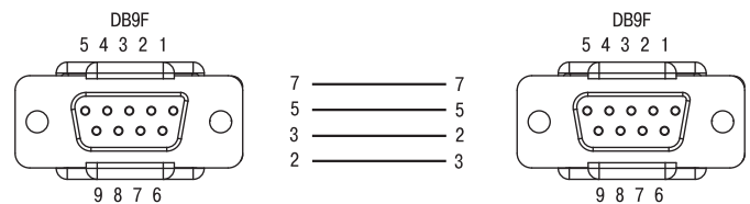
Кабель КС4 для підмикання ПЛК100 до панелей ІП320, СП270 та СП3хх (порт RS-232 Download)
