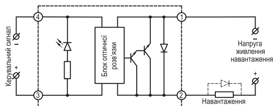
Схема вмикання серії HD-xx25.DD3
