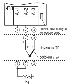
Схема підмикання вхідних сигналів
