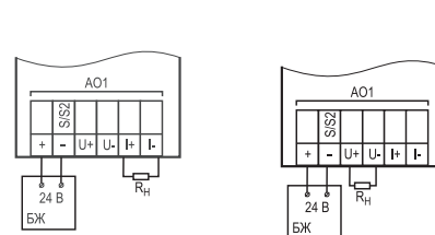
Схема підм'якання навантаження до ВЕ типу И
