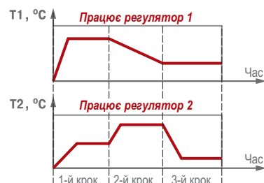
Приклад програми для двоканалного регулятора ТРМ151-01
