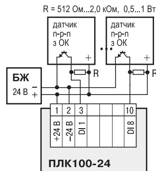
ПЛК100-24, датчик п-р-п-типу
