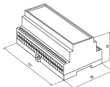
Д9 — корпус для кріплення на DIN-рейку 35 мм, габаритні розміри: 157х86х58 мм, ступінь захисту з боку передньої панелі IP20
