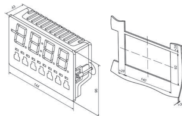
Щ8 — корпус щитового кріплення габаритні розміри: 144х96х43 мм, ступінь захисту: з боку передньої панелі IP54 з боку циліндричної частини корпусу IP20
