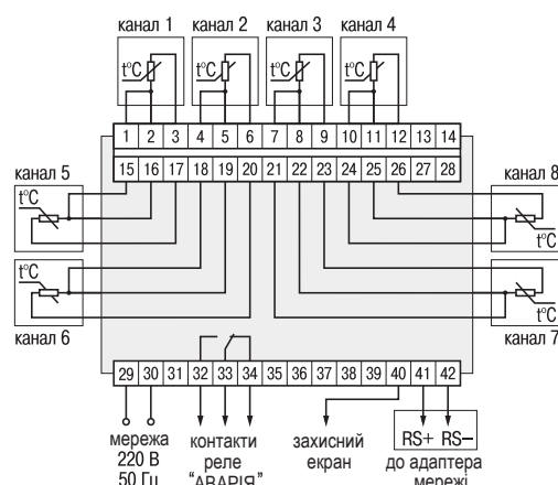
Схема підмикання пристрою модифікації УКТ38-В.01 та УКТ38-В.03 з термоперетворювачами опору типу ТОМ, ТОП
