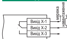
Вихідний елемент типу Р (е/м реле)
