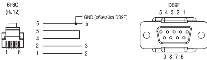
Схема кабелю програмування KC1, що входить до комплексу постачання
