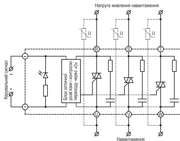
Схема вмикання серії HDH-xx44.ZD3
