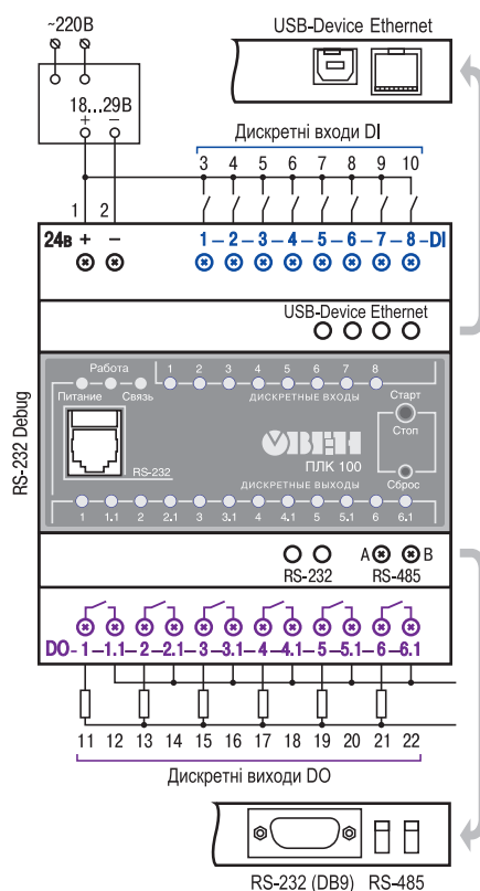
Схема підмикання ПЛК100-24.Р
