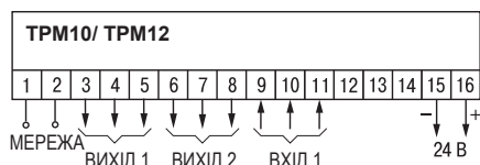
Схема розташування та призначення клем TRM10, TRM12
