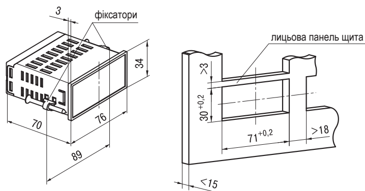
Щ3 — корпус щитового кріплення габаритні розміри: 76х34х70 мм ступінь захисту з боку передньої панелі IP54
