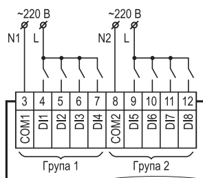
Схема підмикання дискретних входів для змінного струму (~220 В)
