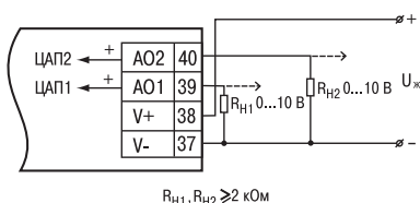
Схема підмикання аналогових виходів типу U PR200-x.4, PR200-220.24
