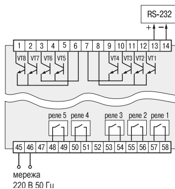
Схема підключення транзисторних ключів та вихідних пристроїв
