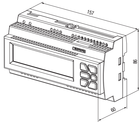
Габаритний кресленник ПЛК63 у корпусі для кріплення на DIN-рейку 35 мм
