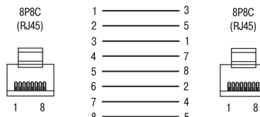
Розведення кабелю для з'єднання ПЛК з комп'ютером по мережі Ethernet напряму
