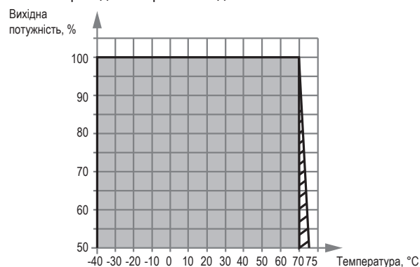
Графік залежності вихідної потужності блоку живлення ( P_{\text{вих}} ) від температури навколишнього середовища ( T_{\text{нав.серед.}} ). БЖ для важких умов експлуатації
