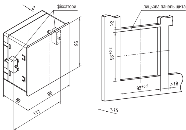
Щ1 — корпус щитового кріплення габаритні розміри: 96х96х65 мм ступінь захисту з боку передньої панелі IP54
