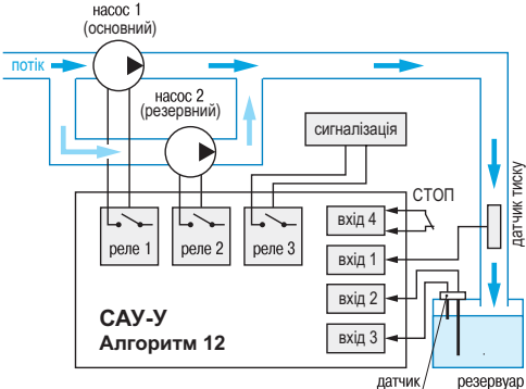
Алгоритм 12 Алгоритм 16
