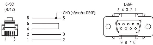
Схема кабелю для програмування КС1, що входить до комплекту постачання
