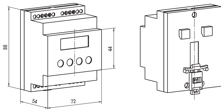
Д — корпус для кріплення на DIN-рейку габаритні розміри: 72х88х54 мм ступінь захисту з боку передньої панелі IP20
