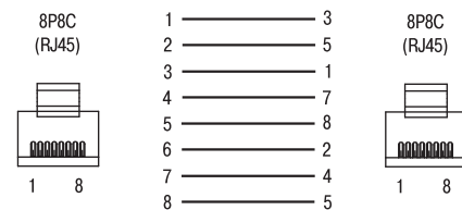
Кабель Ethernet crossover
