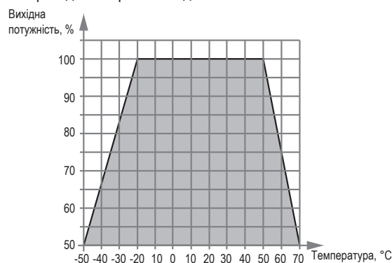
Графік залежності вихідної потужності блоку живлення ( P_{\text{вих}} ) від температури навколишнього середовища ( T_{\text{нав.серед.}} ). БЖ для звичайних умов експлуатації
