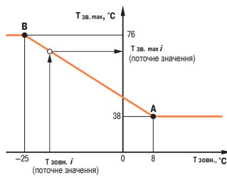
Приклад графіка температури зворотної води — T_{зв.мах.} = f(T_{зовн.})
