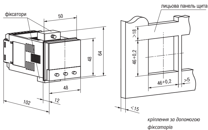
Щ5 — корпус щитового кріплення габаритні розміри: 48х48х102 мм ступінь захисту з боку передньої панелі IP54
